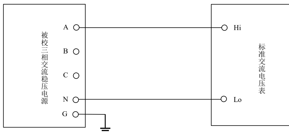
图1 交流电压校准接线图（空载条件）
